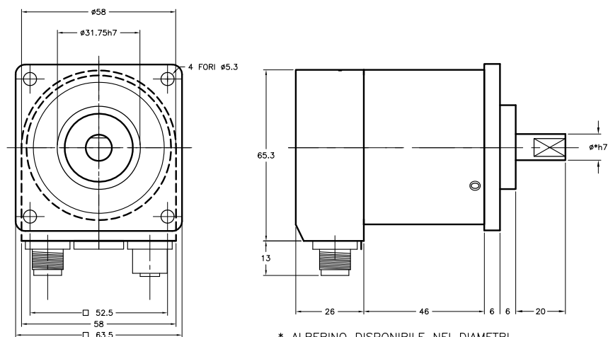
MEM620Bus
