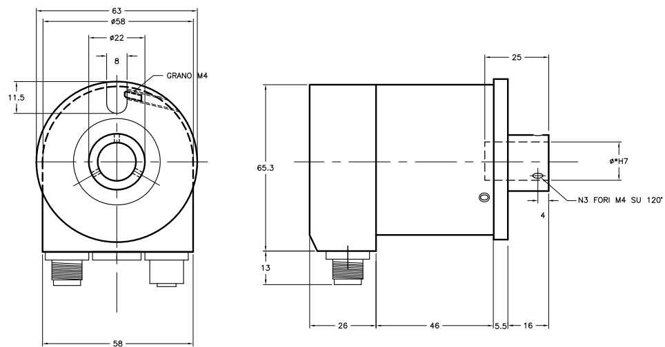
MEM410Bus
